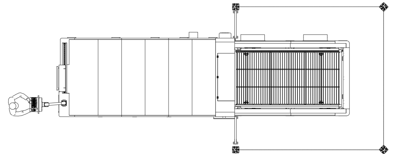
Abbildung mit Lichtschranken zur Absicherung des Laserbereichs; alternativ auch Integration eines Flächenscanners möglich (Verbesserung der Zugänglichkeit der Anlage)
